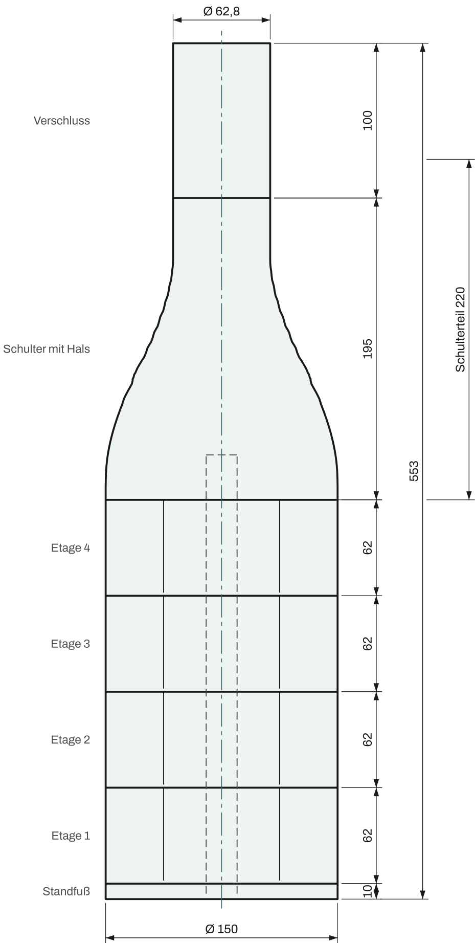
VORDERANSICHT 1 : 2,5
